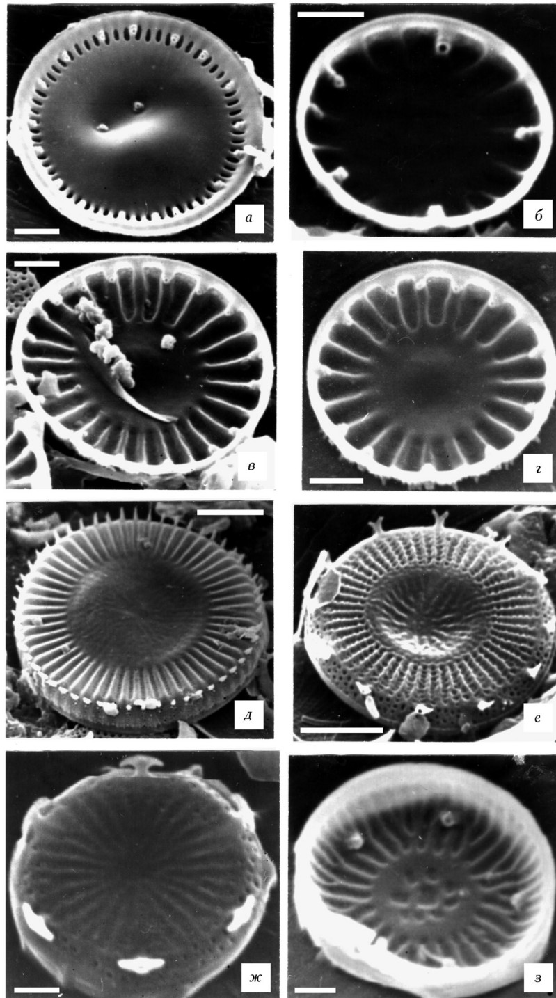
3. Электронные микрофотографии створок (СЭМ): 1 — Cyclotella choctawatcheeana ; 2 — C. marina ; 3, 4 — C. meduanae ; 5 — C. meneghiniana ; 6—8 — Discostella pseudostelligera . 1—4, 8 — створки с внутренней поверхности; 5—7 — створки с наружной поверхности. Масштаб: 1, 3, 4 — 2 мкм; 2, 7, 8 — 1 мкм; 5 — 10 мкм; 6 — 5 мкм.
